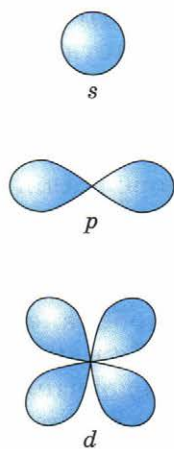
Рис. 3. Формы s -, p -, d -электронных облаков
