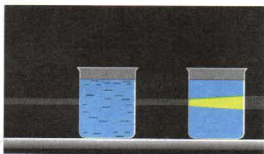
Рис. 87. Эффект Тиндаля
