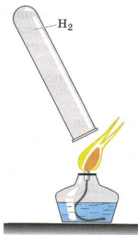
Рис. 54. Проверка водорода на чистоту
