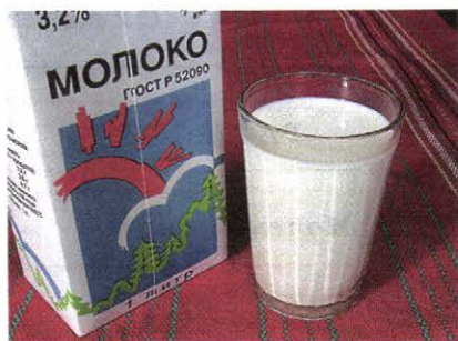
Рис. 80. Природные эмульсии: а — молоко; б — нефть
