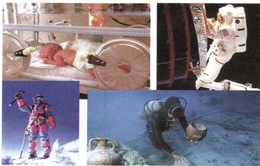
Рис. 57. Кислород необходим для дыхания
