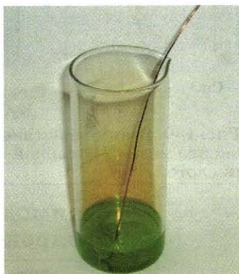
Рис. 128. Взаимодействие концентрированной азотной кислоты с медью сопровождается образованием бурого газа — оксида азота (IV)
