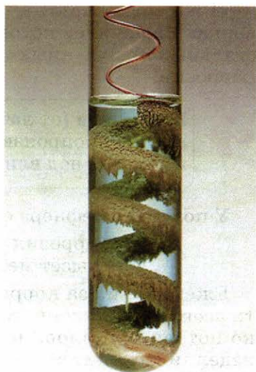
Рис. 120. Взаимодействие меди с раствором нитрата серебра
