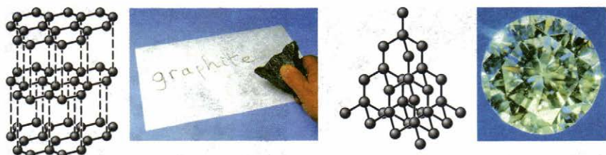
Рис. 92. Графит и алмаз — две аллотропные модификации углерода
