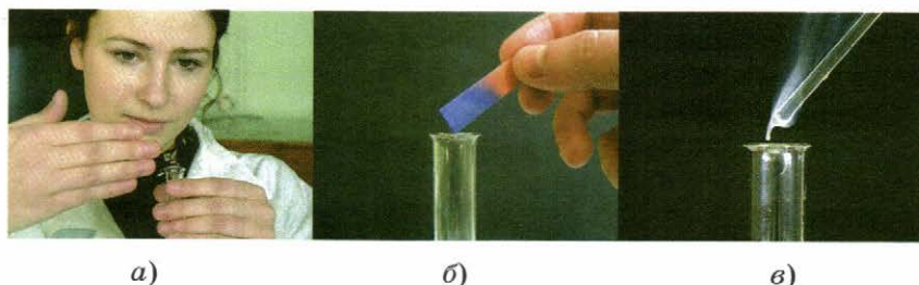
Рис. 65. Распознавание аммиака: а — по запаху; б — по изменению окраски индикаторной бумажки; в — по появлению дыма при поднесении стеклянной палочки, смоченной соляной кислотой
