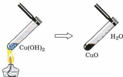
Рис. 136. Разложение гидроксида меди (II) при нагревании
