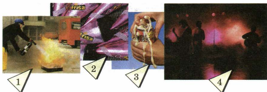
Рис. 61. Применение углекислого газа: 1 — тушение пожаров; 2 — хранение мороженого; 3 — производство шипучих напитков; 4 — создание спецэффектов на сцене
