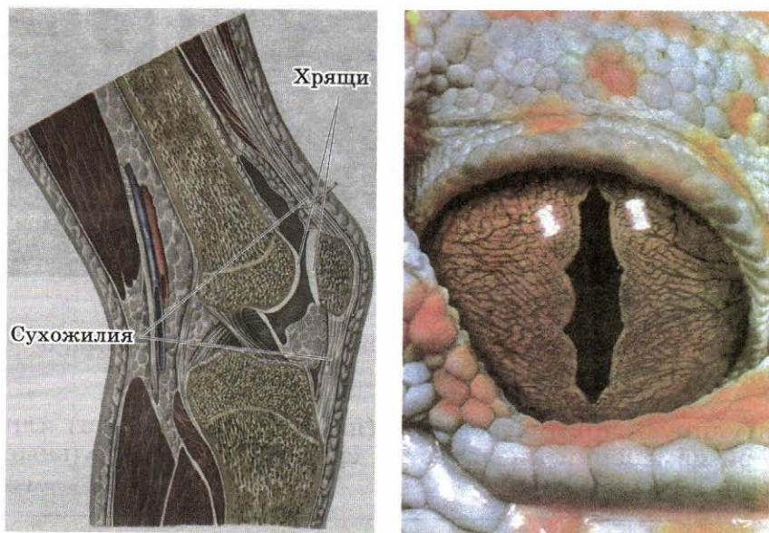
Рис. 85. Коллоидные системы в живых организмах
