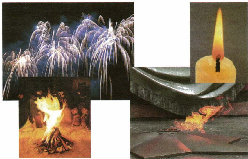
Рис. 58. Кислород поддерживает горение
