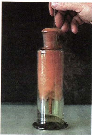
Рис. 116. Взаимодействие железа с хлором
