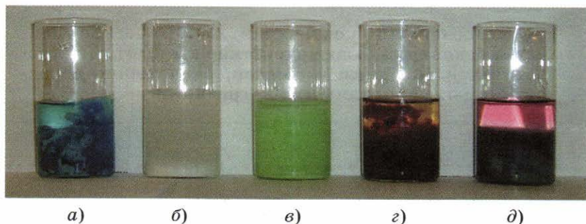
Рис. 135. Нерастворимые гидроксиды, полученные реакцией обмена: a — гидроксид меди (II); б — гидроксид магния; в — гидроксид никеля (II); г — гидроксид железа (III); д — гидроксид кобальта (II)
