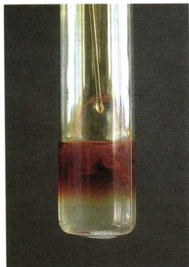
Рис. 125. Вытеснение брома из его соли более активным галогеном
