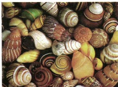
Рис. 142. Раковины состоят из карбоната кальция
