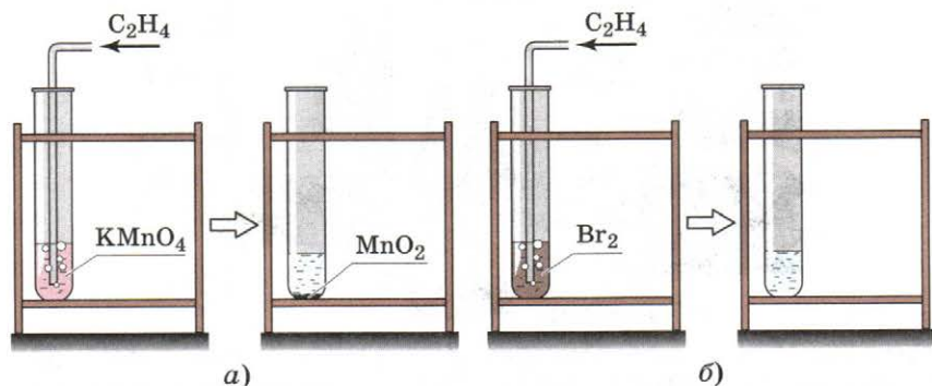
Рис. 68. Распознавание этилена с использованием: а — раствора перманганата калия; б — бромной воды
