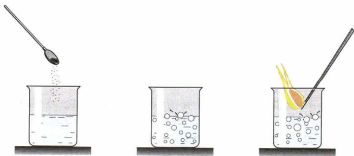
Рис. 105. Разложение пероксида водорода с использованием оксида марганца (IV)
