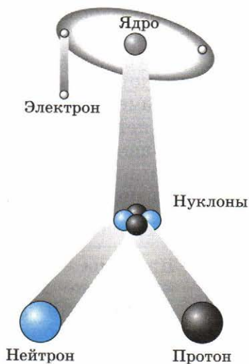
Рис. 2. Схема строения атома
