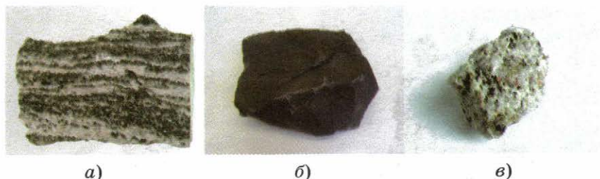
Рис. 23. Природные сплавы: а — гнейс; б — базальт; в — гранит
