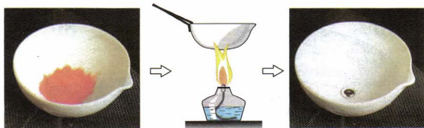
Рис. 94. Получение кислорода разложением оксида ртути
