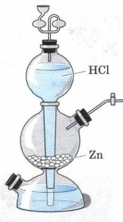
Рис. 53. Аппарат Киппа
